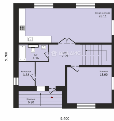
План 1 этажа
